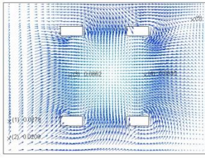
図14 風速1 風速分布 (高さ 1.4m)
