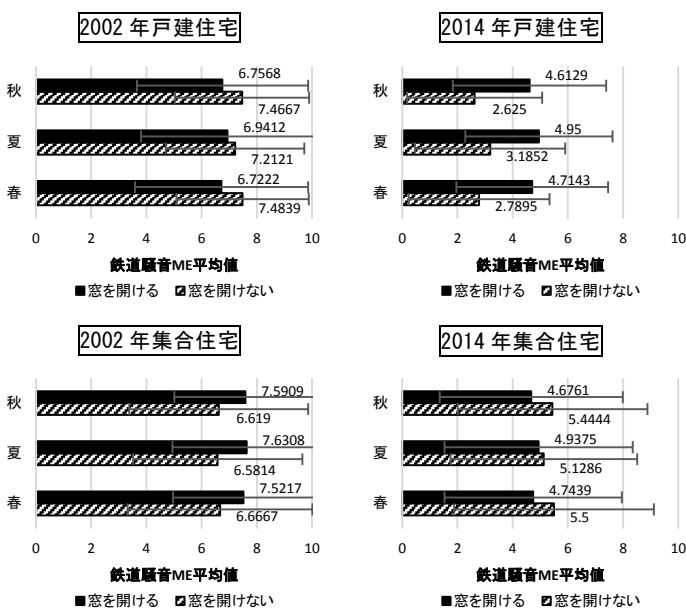
図 5.7.1 居間での窓開放程度と鉄道騒音 ME 平均値の関係
