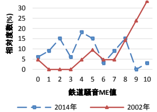
図 8.2.2-1 東側かつ居住階が高架化前後の比較 p<.0001
