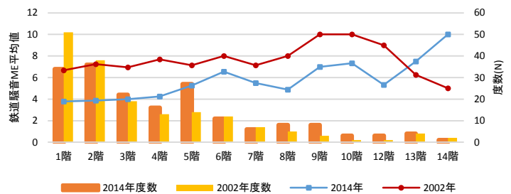
図 8.1.1 居住階毎の鉄道騒音 ME 平均値の比較
