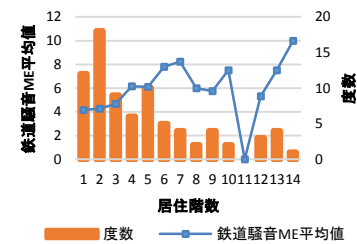
図 8.2.1-2 西側のみ居住階毎の鉄道騒音 ME 平均値
