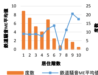
図 8.2.1-1 東側のみ居住階毎の鉄道騒音 ME 平均値
